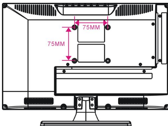
Retro della TV
