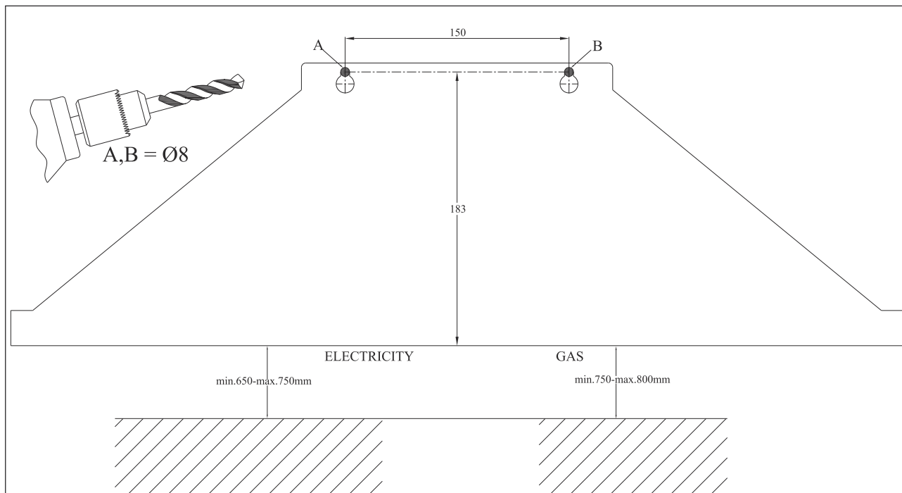
Fig. 8: 2240 MONTAJ ŞABLONU
