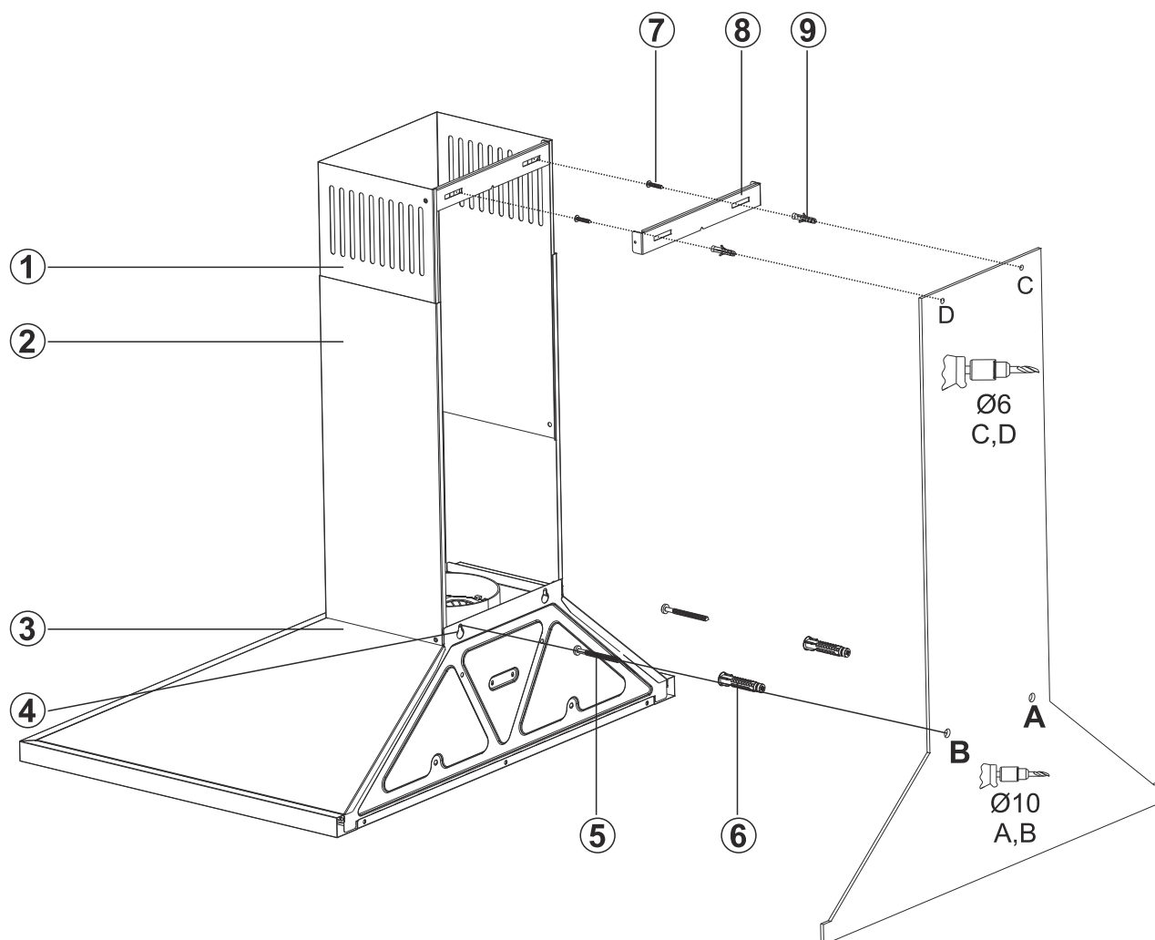
Fig. 12: INSTALLAZIONE E PARTI
