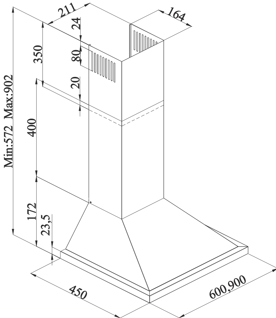
Fig. 1: 2240 60_90 ÇİFT BACA TEKNİK ÇİZİM
