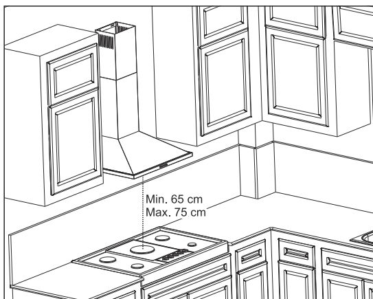
Fig. 7: INSTALLAZIONE DELL'APPARECCHIATURA
