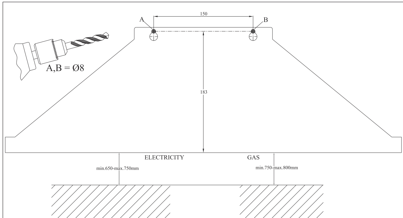
Fig. 8: 2240 MONTAJ ŞABLONU
