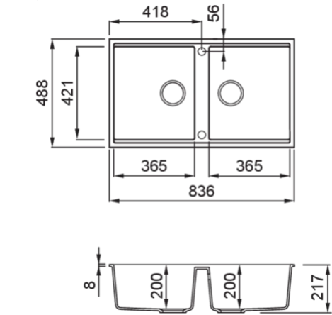
Disegno tecnico
