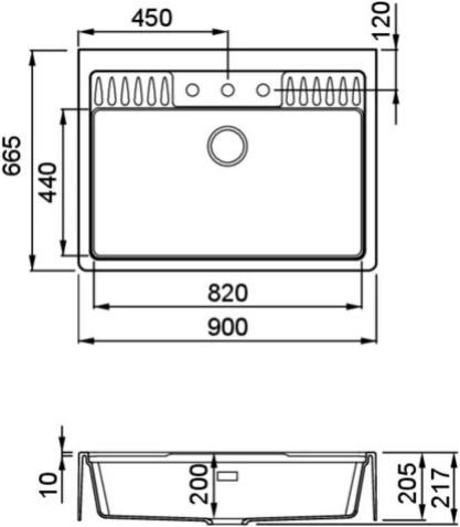
Disegno tecnico
