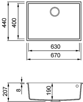
Disegno tecnico
