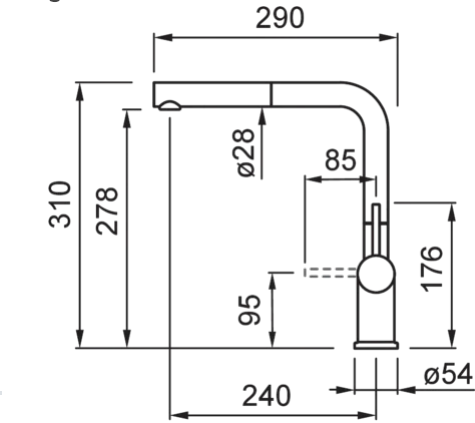
Disegno tecnico
