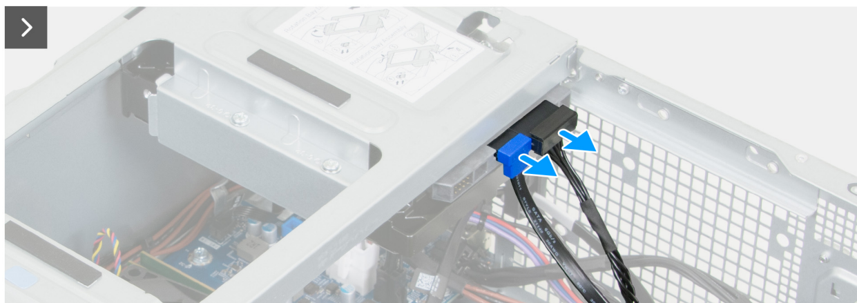
Figura 28. Rimozione del drive bay
