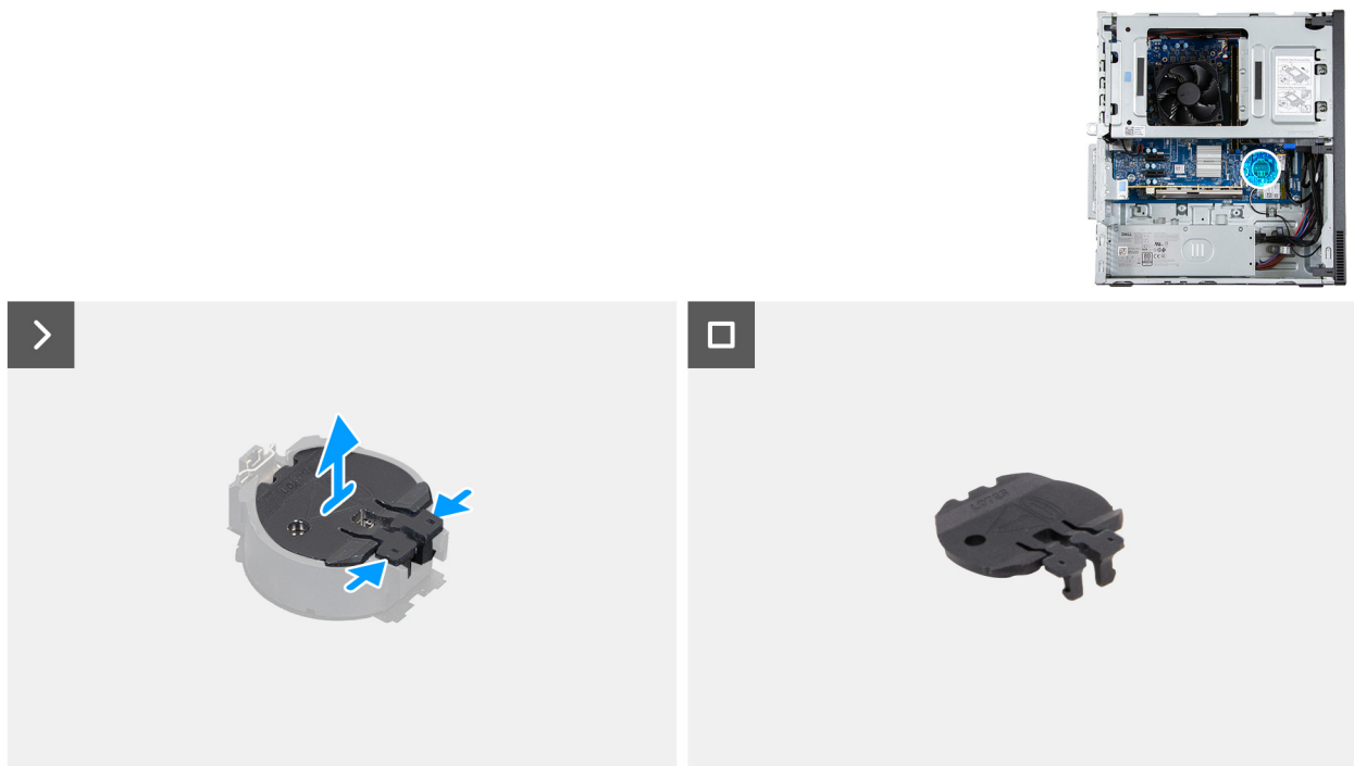
Figura 14. Rimozione del coperchio della batteria a bottone
