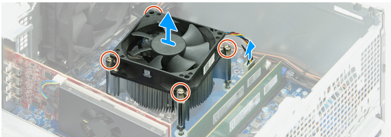
Figura 50. Rimozione del gruppo ventola del processore e dissipatore di calore
