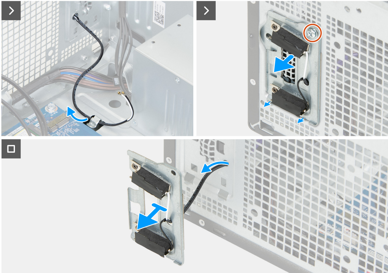
Figura 44. Rimozione dei moduli dell'antenna
