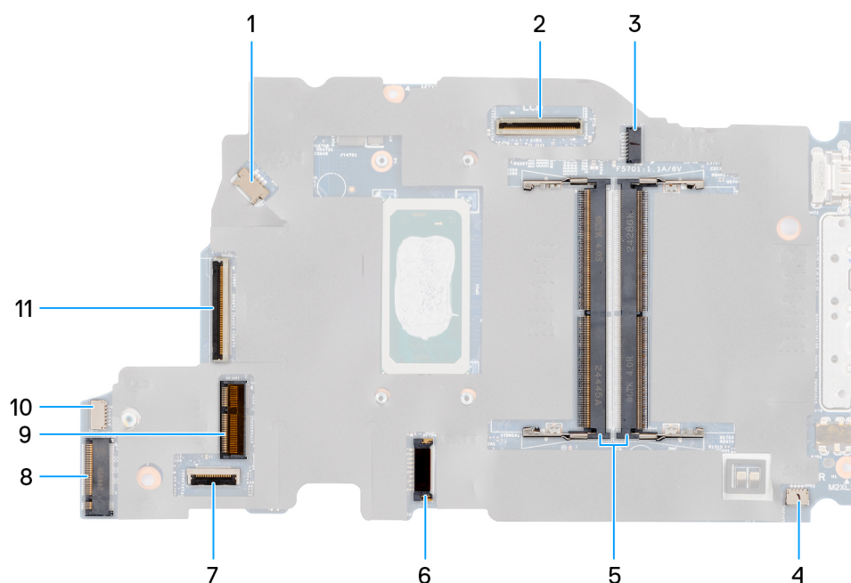
Figura 63. Connettori scheda di sistema
