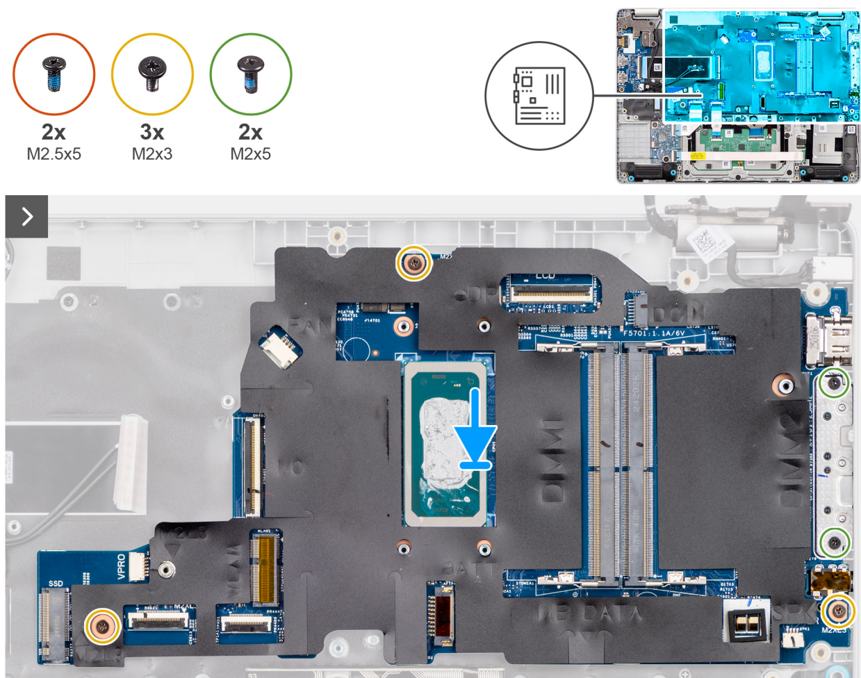
Figura 73. Installazione della scheda di sistema
