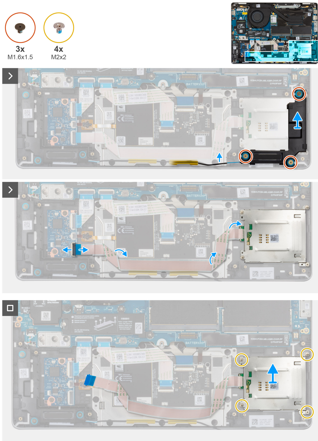
Figura 48. Rimozione del lettore di smart card
