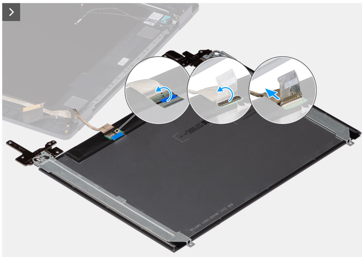
Figura 113. Rimozione del gruppo del pannello del display
