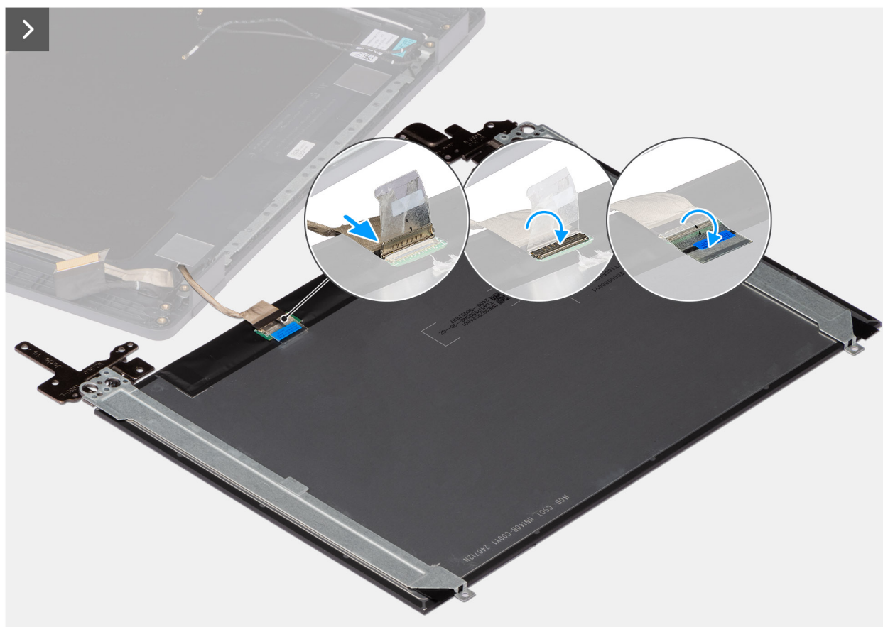
Figura 116. Installazione del gruppo del pannello del display
