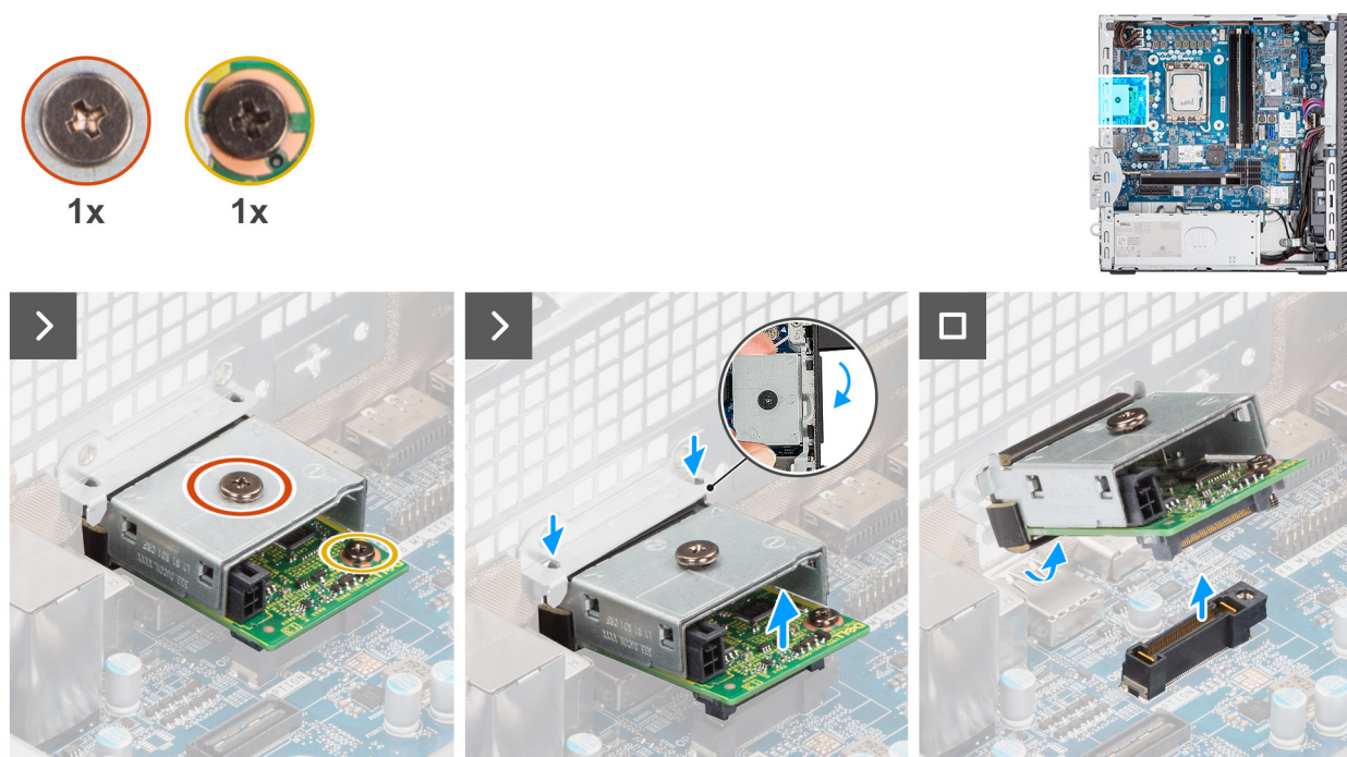
Figura 64. Rimozione del modulo USB opzionale
