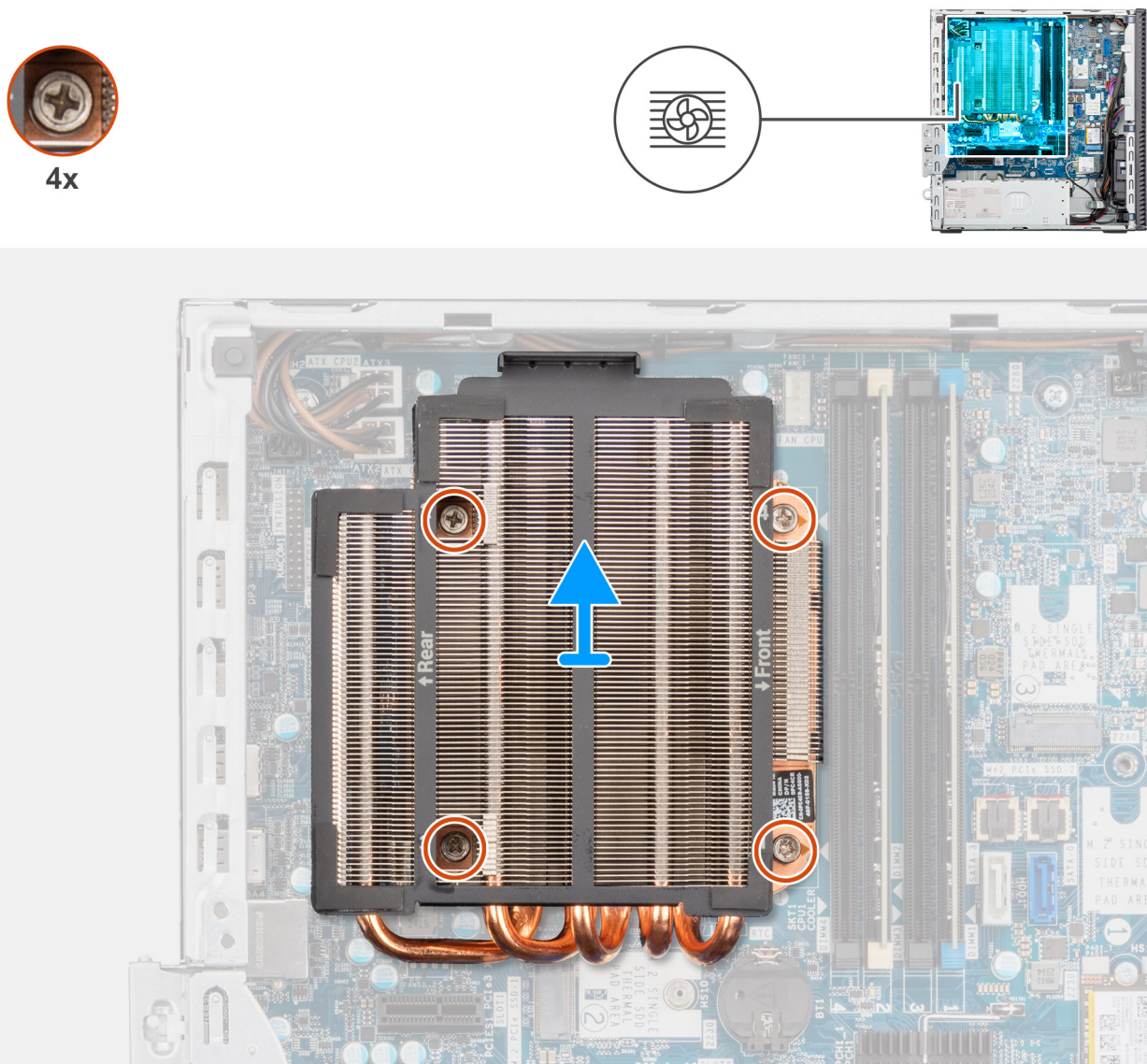
Figura 53. Rimozione del gruppo del dissipatore di calore del processore
