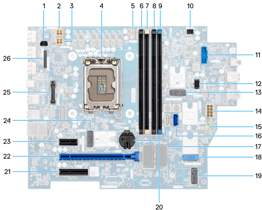
Figura 87. Panoramica della scheda di sistema
