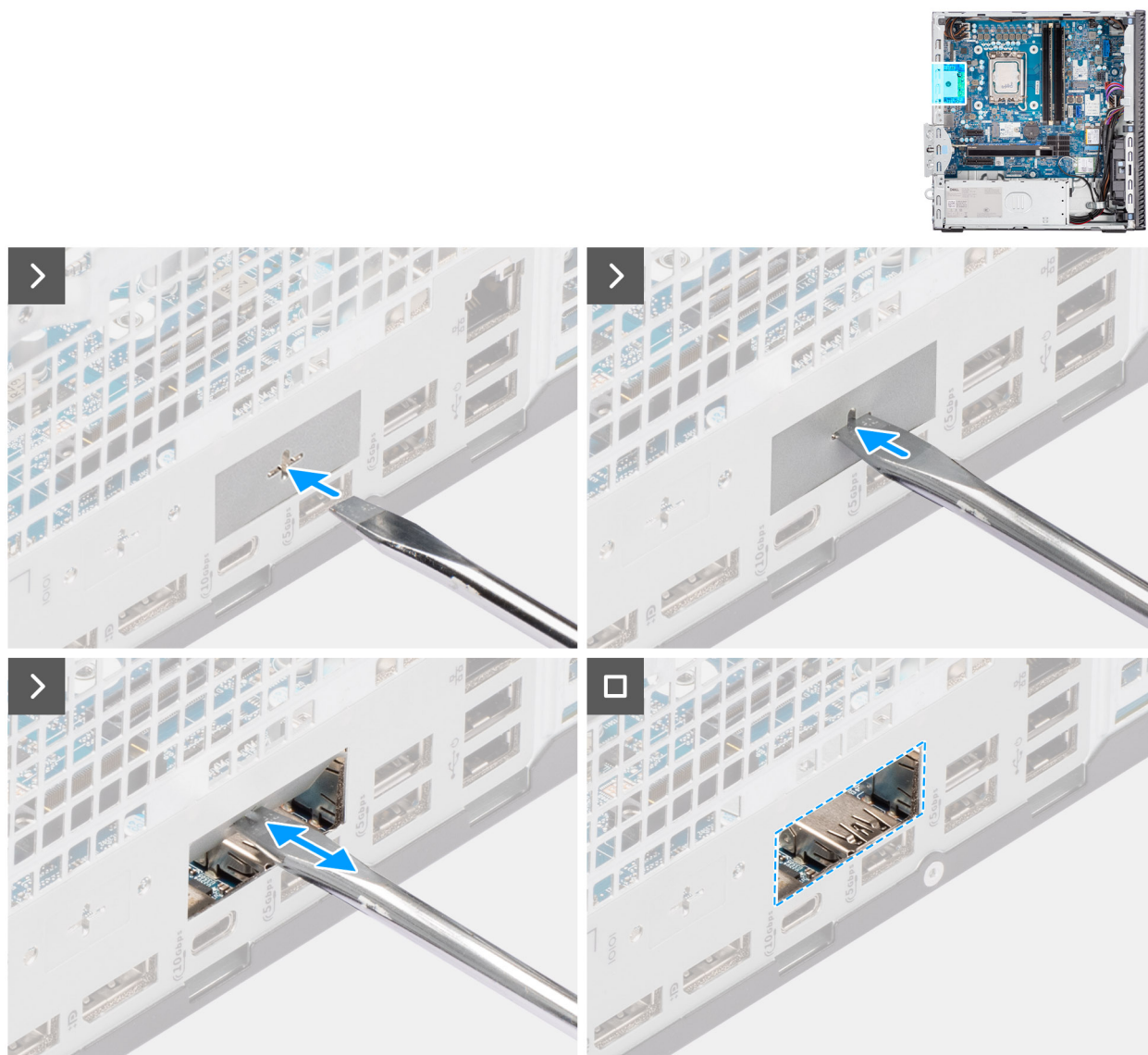
Figura 77. Installare il modulo DisplayPort opzionale.
