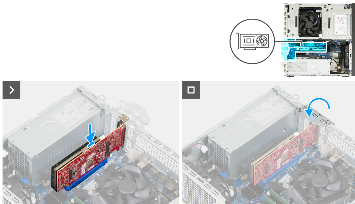
Figura 40. Installazione della scheda grafica
