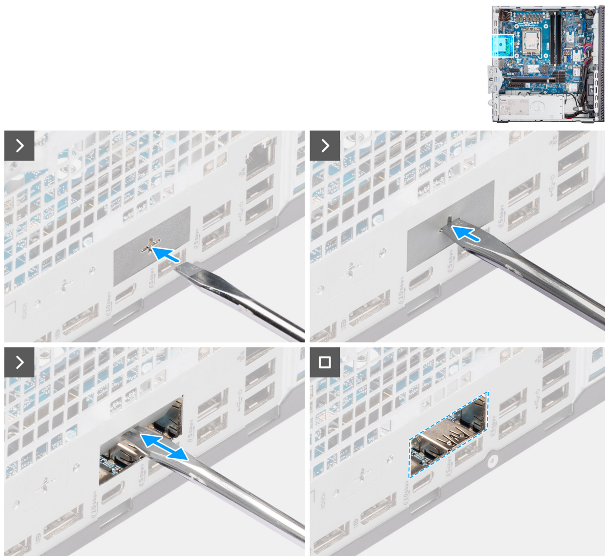
Figura 68. Installazione del modulo Thunderbolt opzionale
