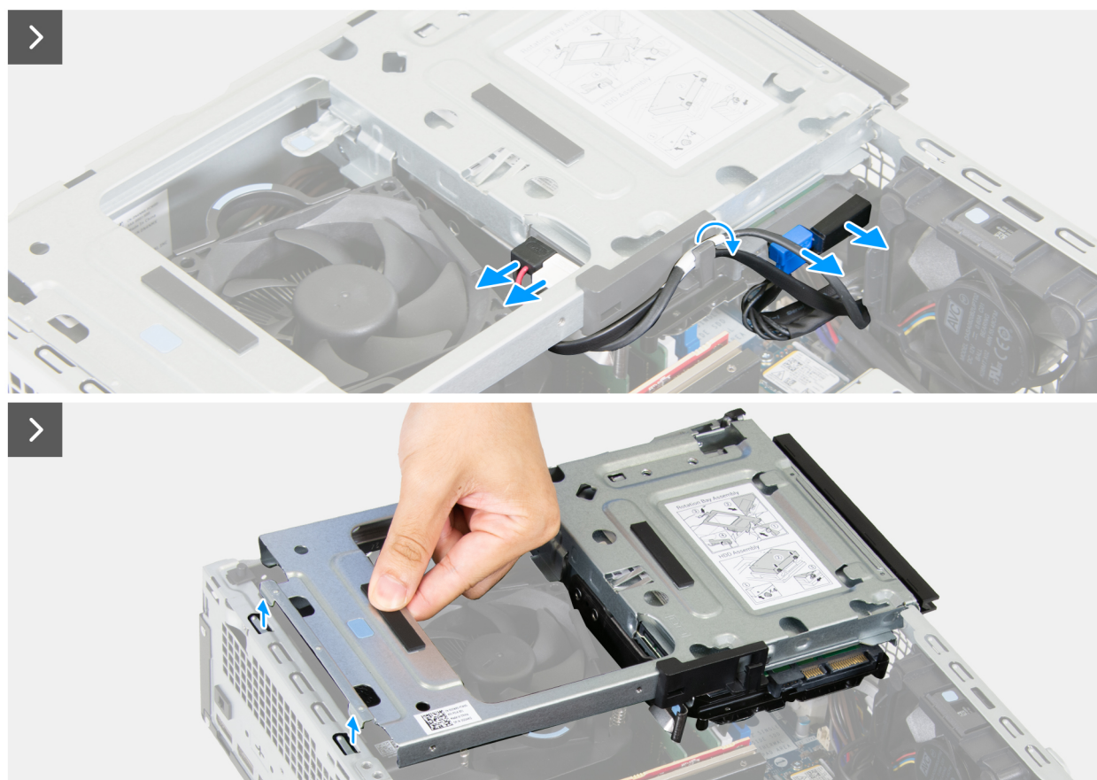
Figura 21. Rimozione del drive bay
