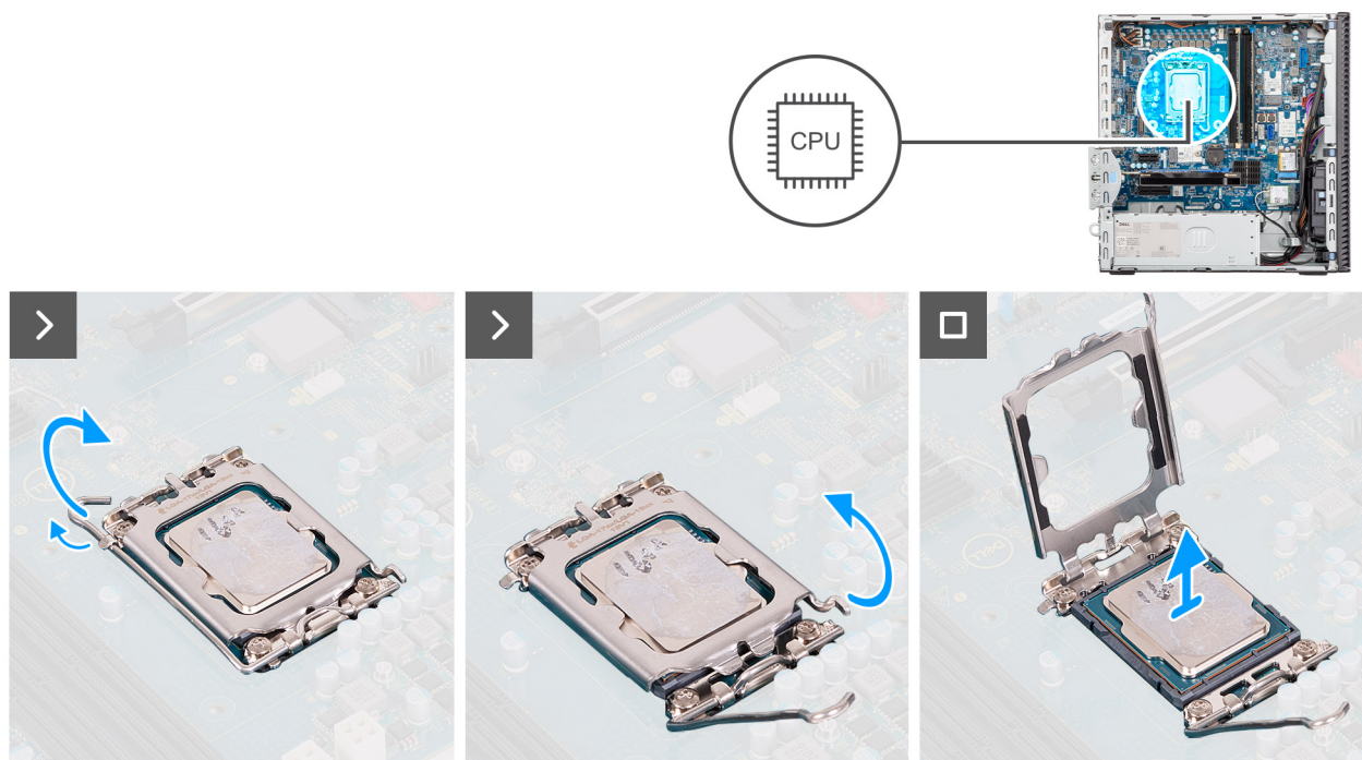
Figura 55. Rimozione del processore
