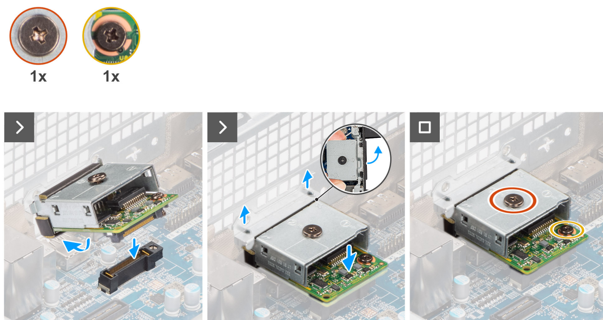
Figura 72. Installare il modulo LAN opzionale.
