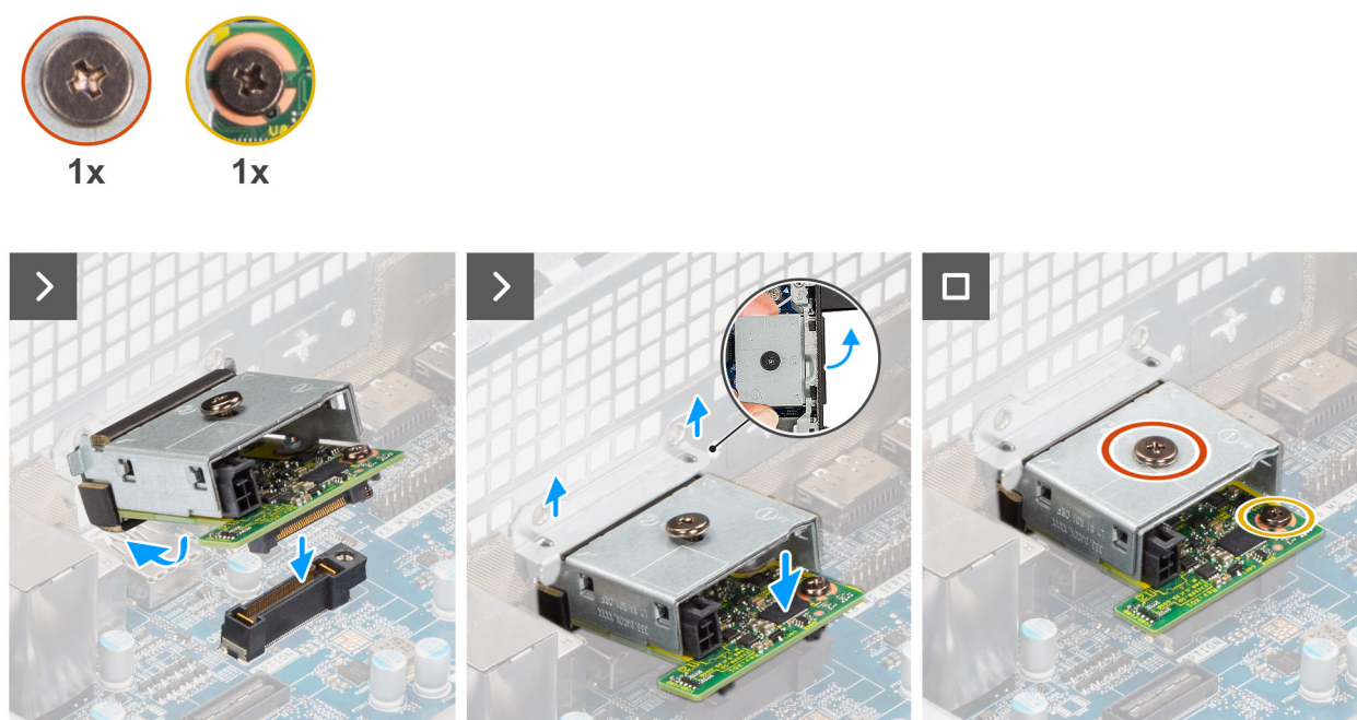
Figura 69. Installazione del modulo Thunderbolt opzionale
