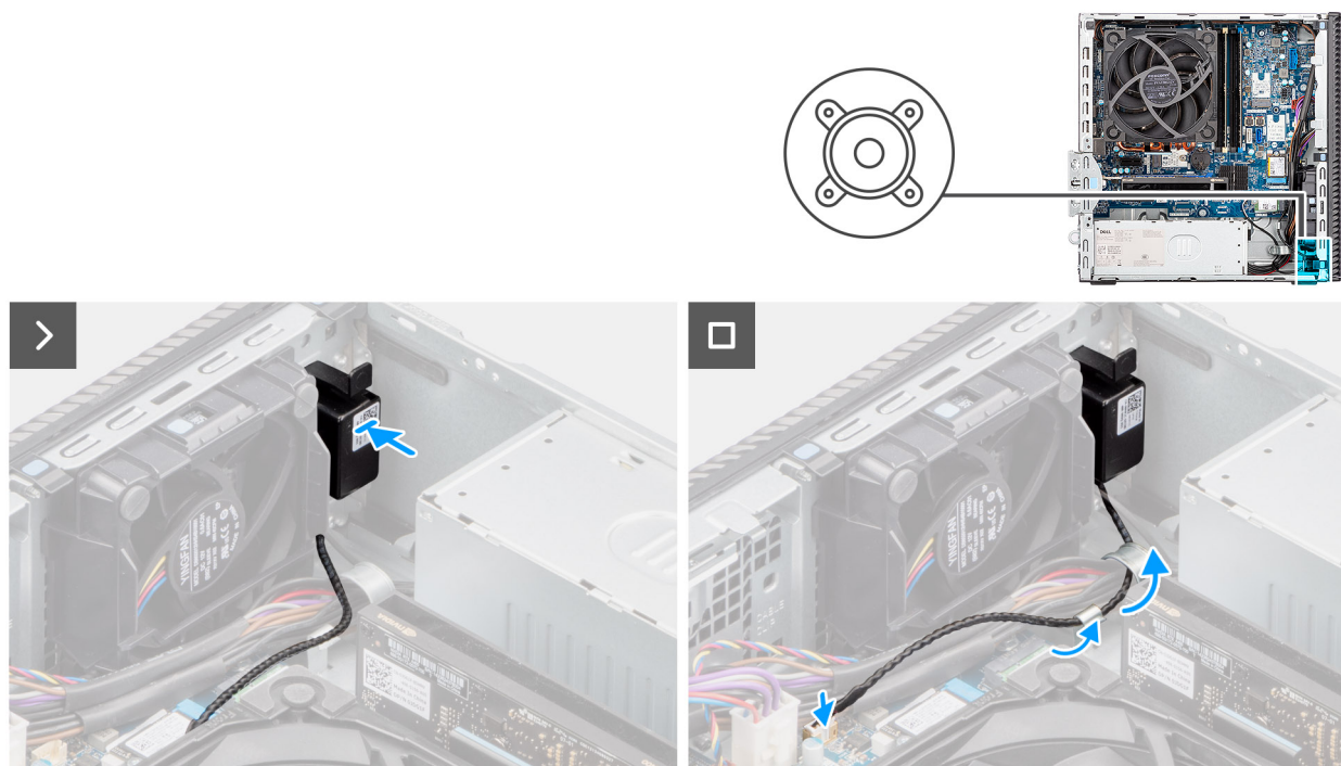
Figura 26. Installazione dell'altoparlante interno
