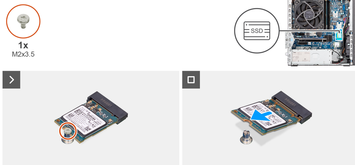
Figura 31. Rimozione dell'unità SSD M.2 2230
