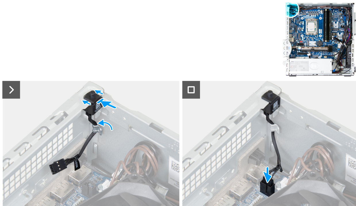
Figura 44. Installazione dello switch antintrusione
