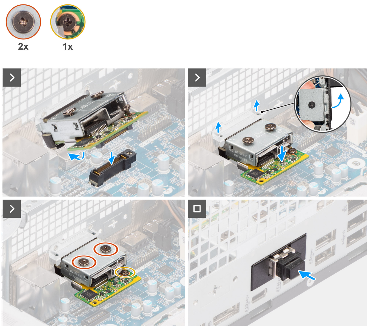
Figura 81. Installazione del modulo ottico opzionale da 5GbE
