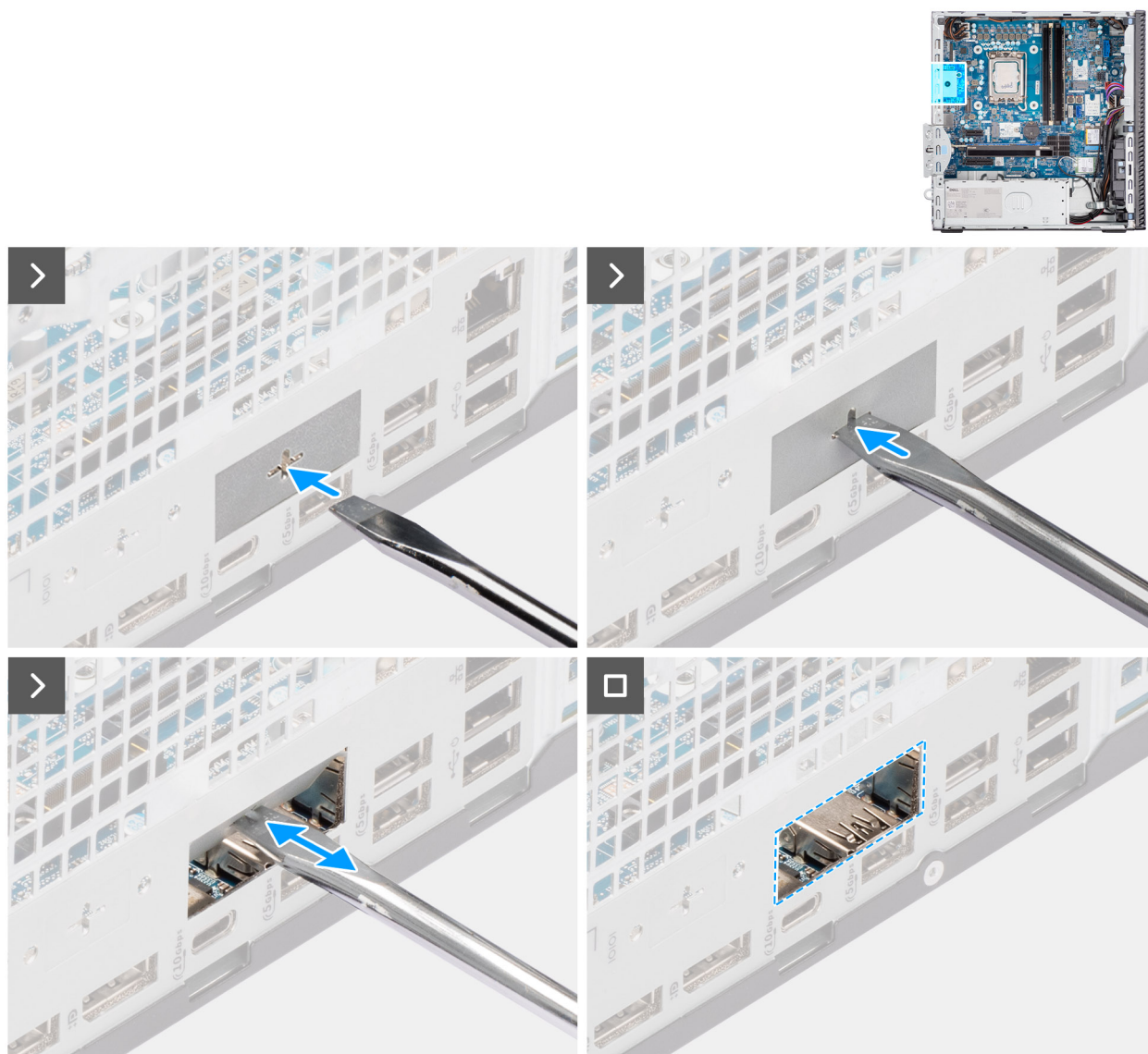
Figura 74. Installare il modulo HDMI opzionale.
