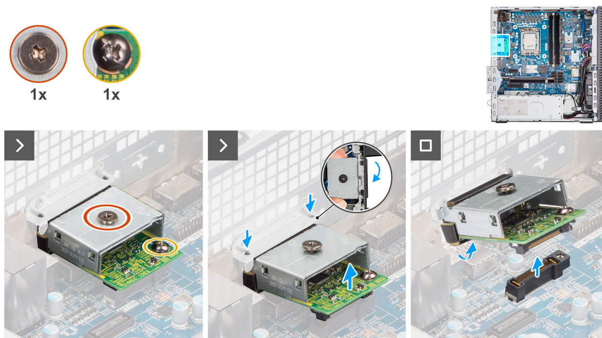
Figura 76. Rimozione del modulo DisplayPort opzionale
