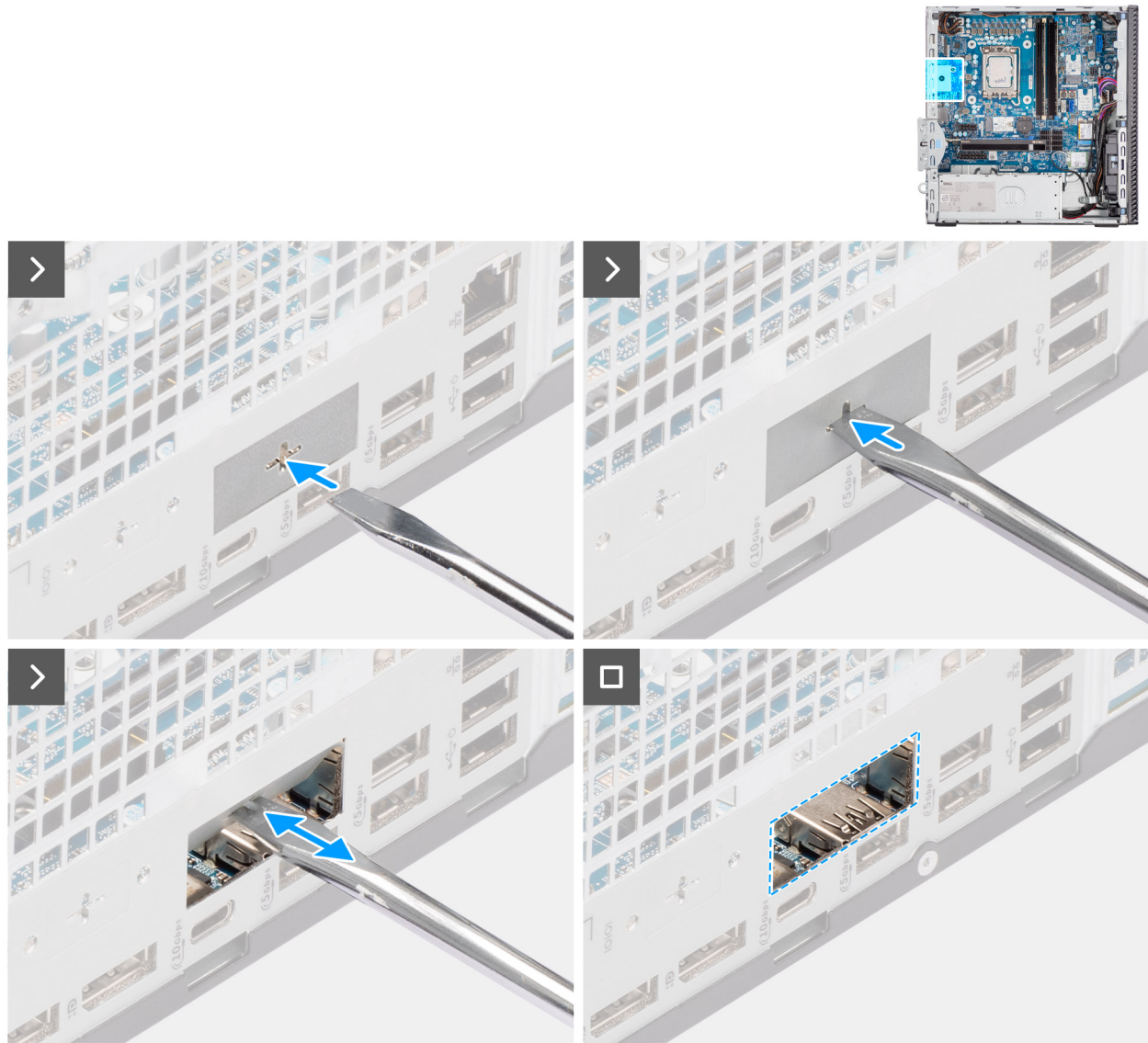
Figura 62. Installare il modulo VGA opzionale.
