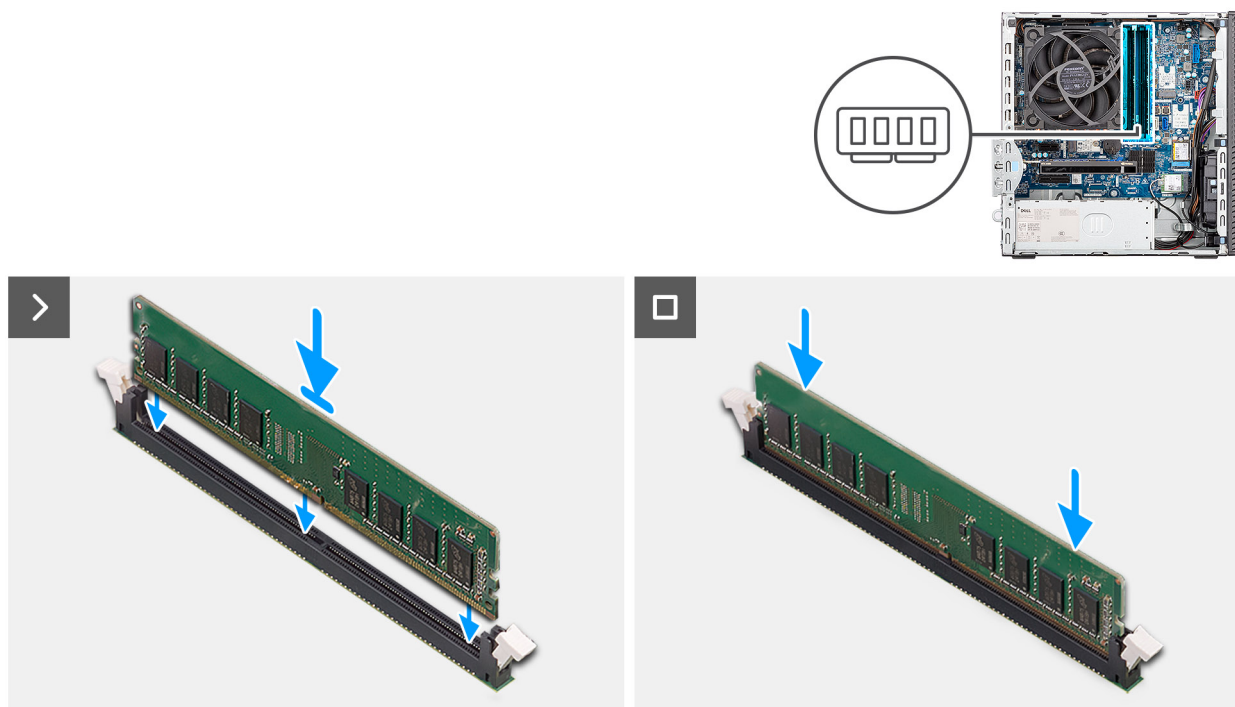
Figura 28. Installazione del modulo di memoria
