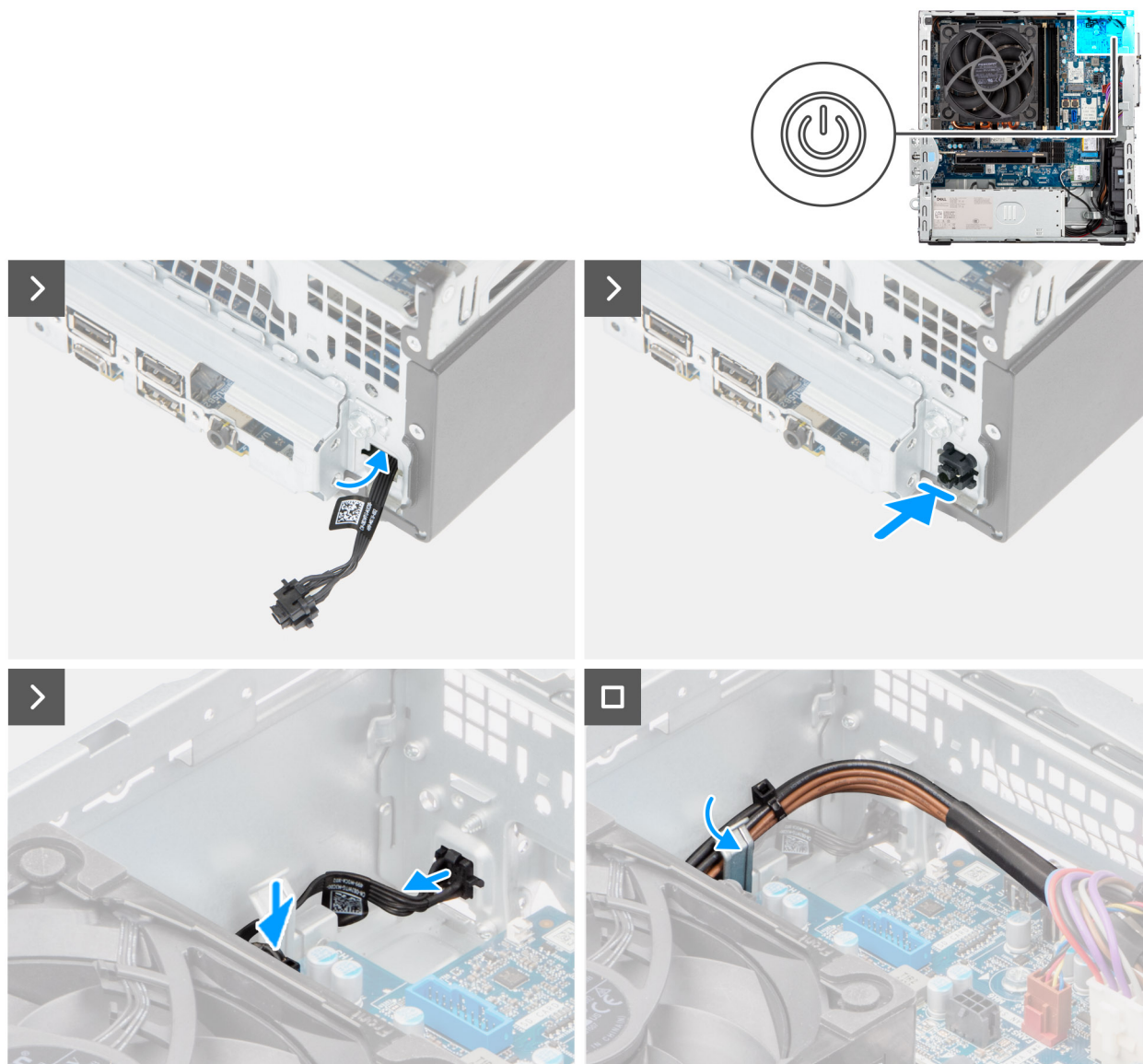
Figura 46. Installazione del pulsante di accensione
