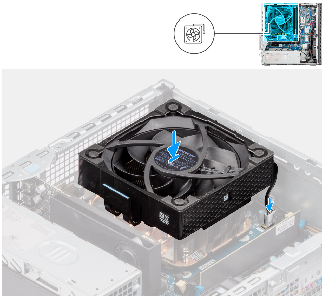
Figura 52. Installazione della ventola del processore
