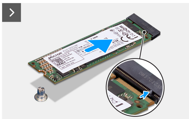
Figura 36. Installazione dell'unità SSD M.2 2280
