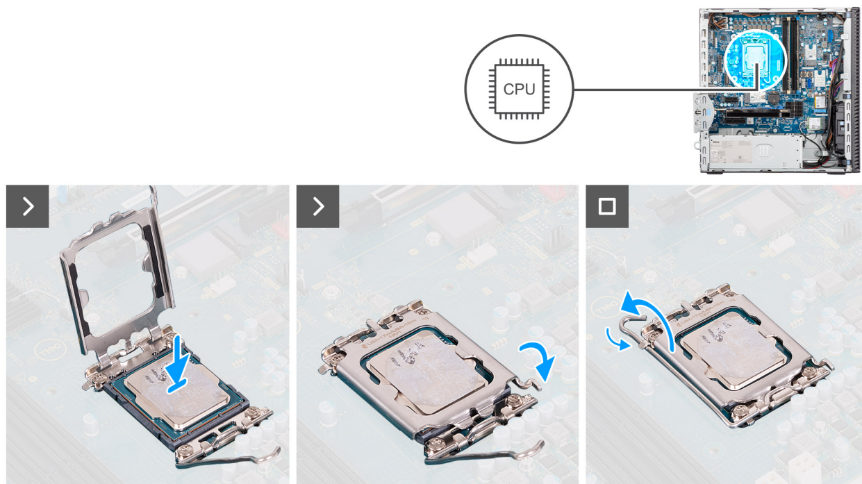
Figura 56. Installazione del processore
