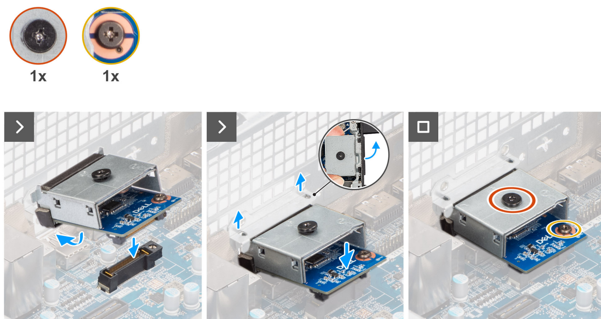
Figura 75. Installare il modulo HDMI opzionale.
