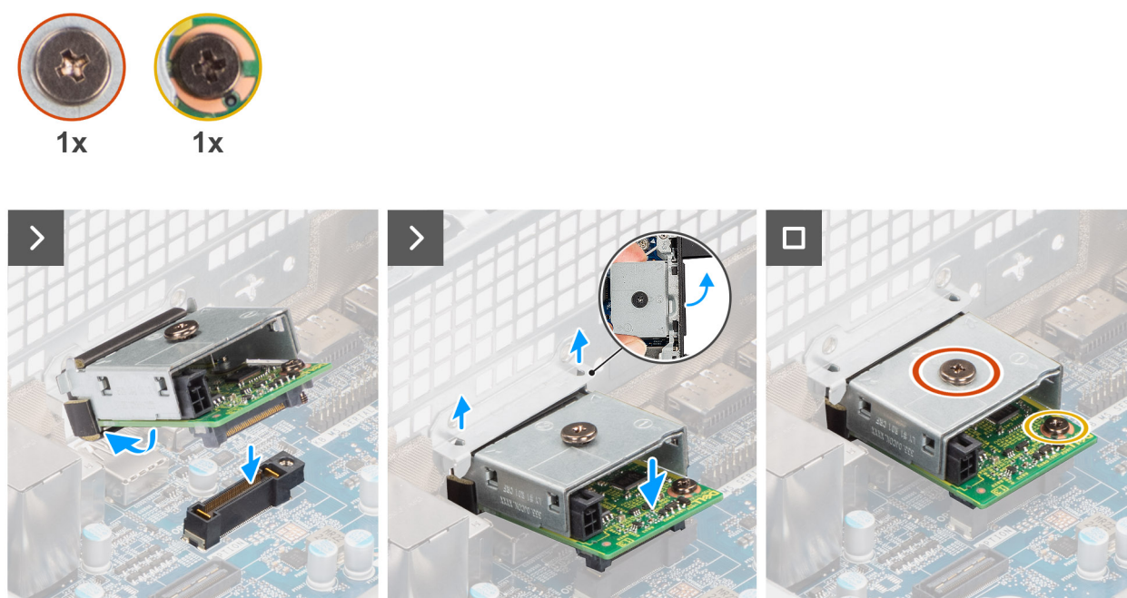
Figura 66. Installare il modulo USB opzionale.
