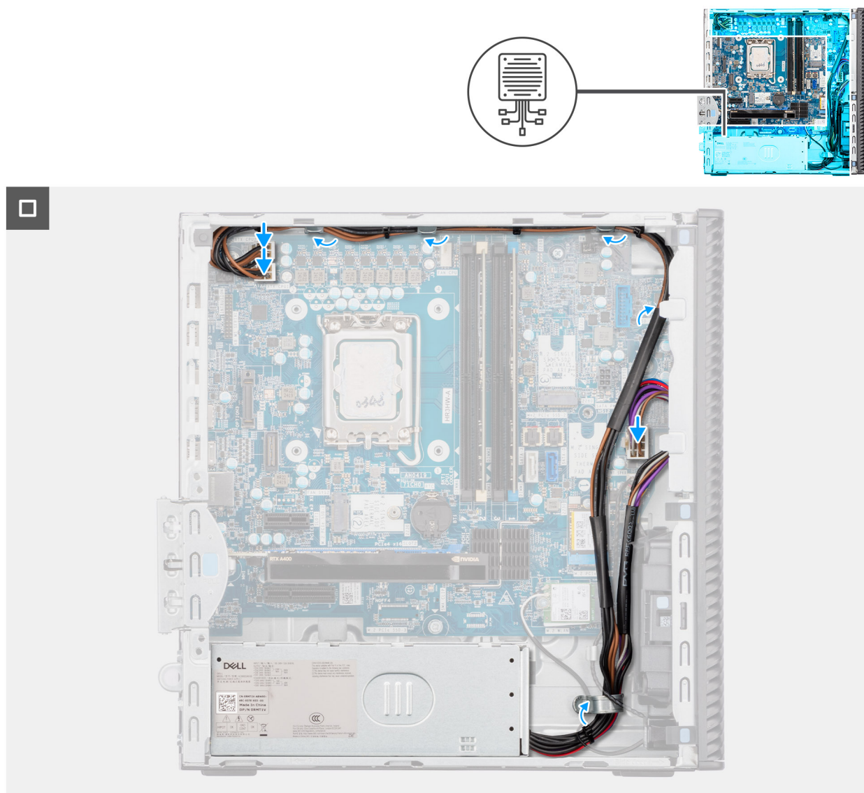
Figura 60. Installazione dell'unità di alimentazione
