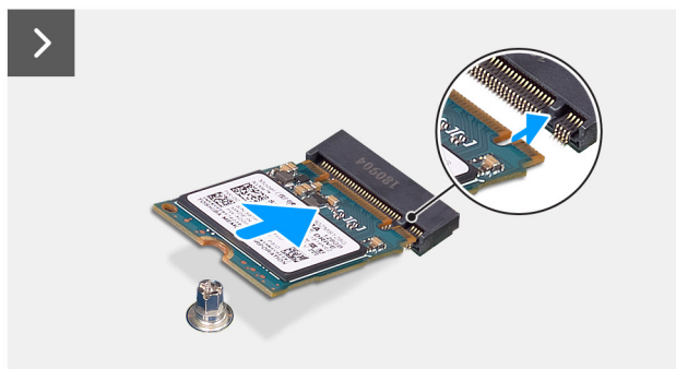
Figura 32. Installazione dell'unità SSD M.2 2230 nello slot 0
