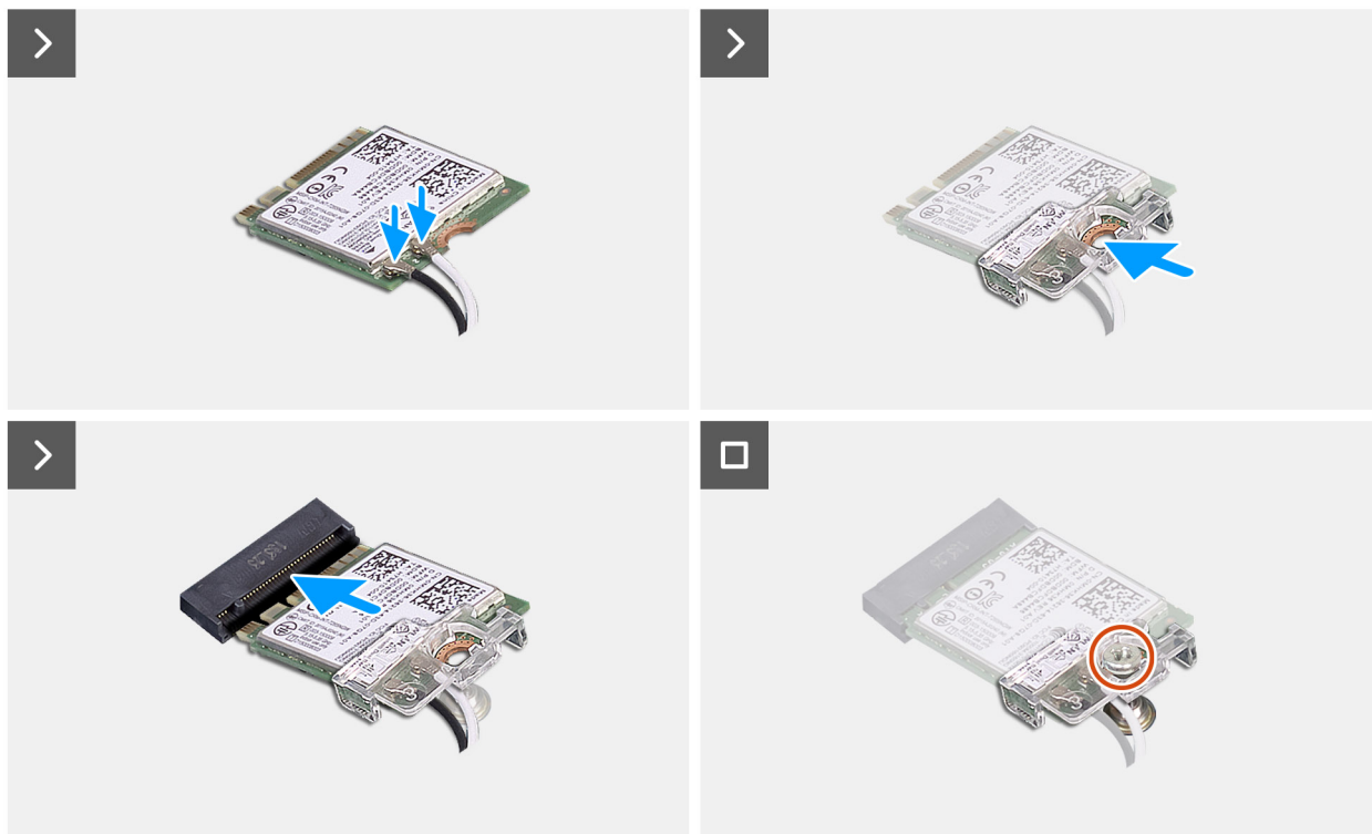
Figura 42. Installazione della scheda wireless
