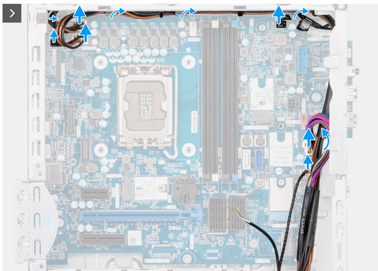
Figura 84. Rimozione della scheda di sistema
