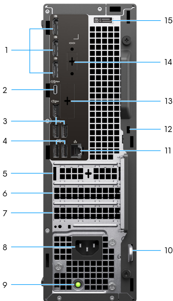
Figura 2. Vista posteriore di Dell Pro Max Slim FCS1250
