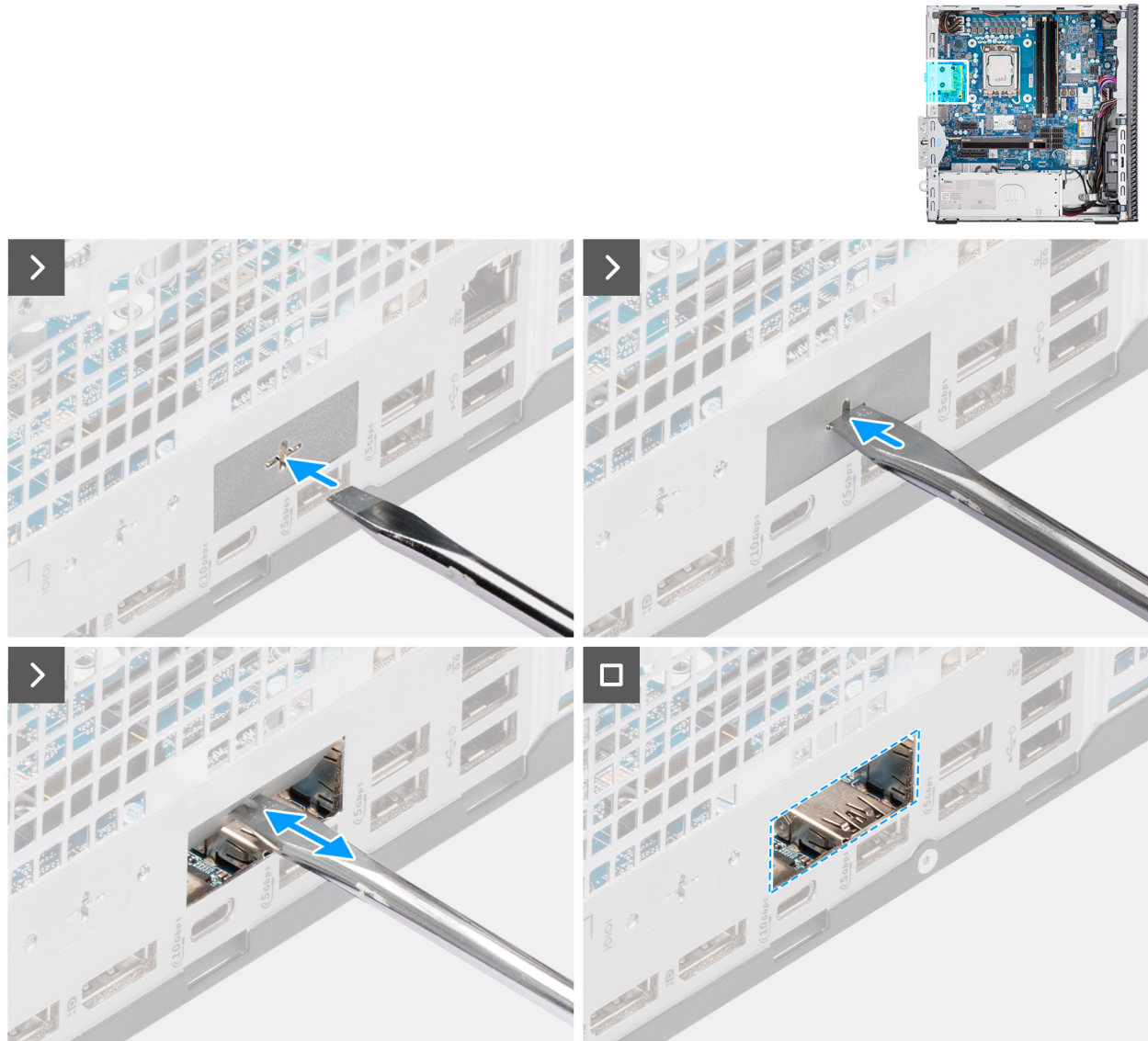
Figura 80. Installazione del modulo ottico opzionale da 5GbE
