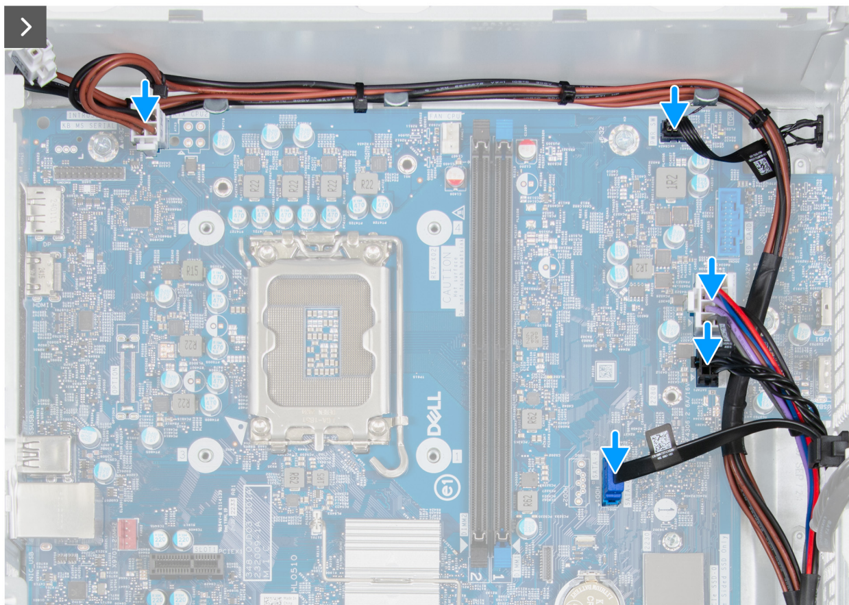
Figura 62. Installazione della scheda di sistema
