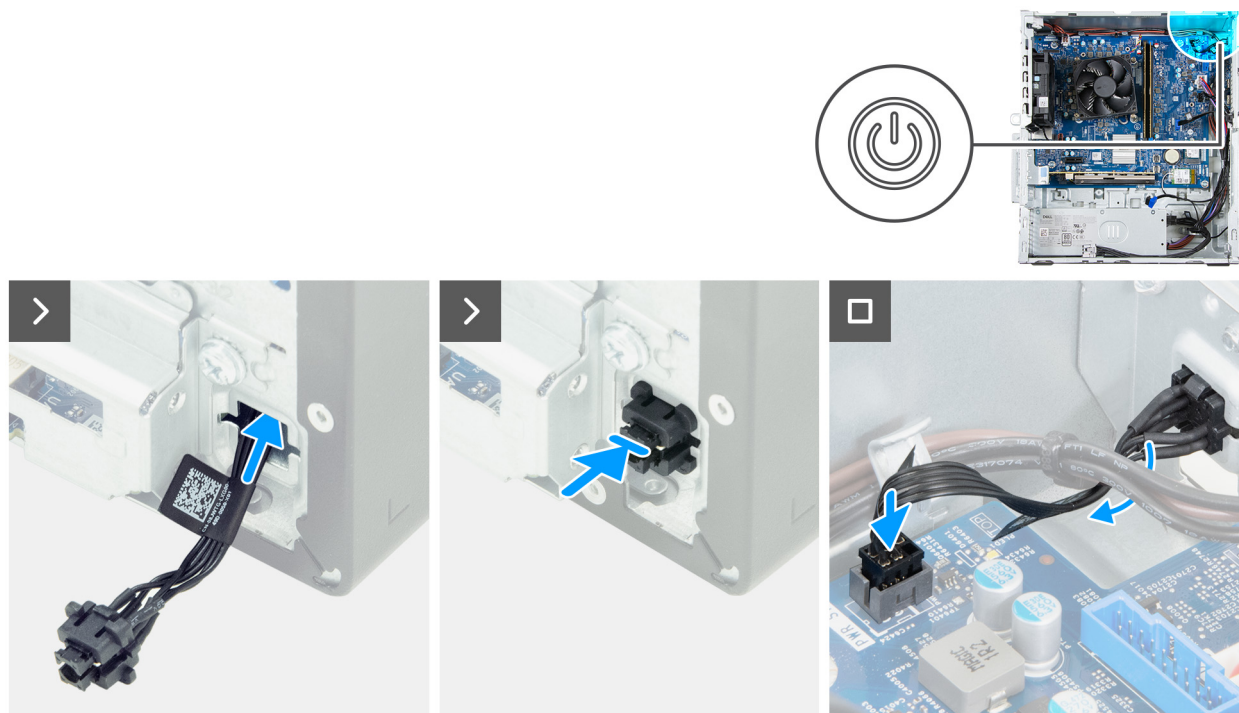
Figura 36. Installazione del pulsante di accensione
