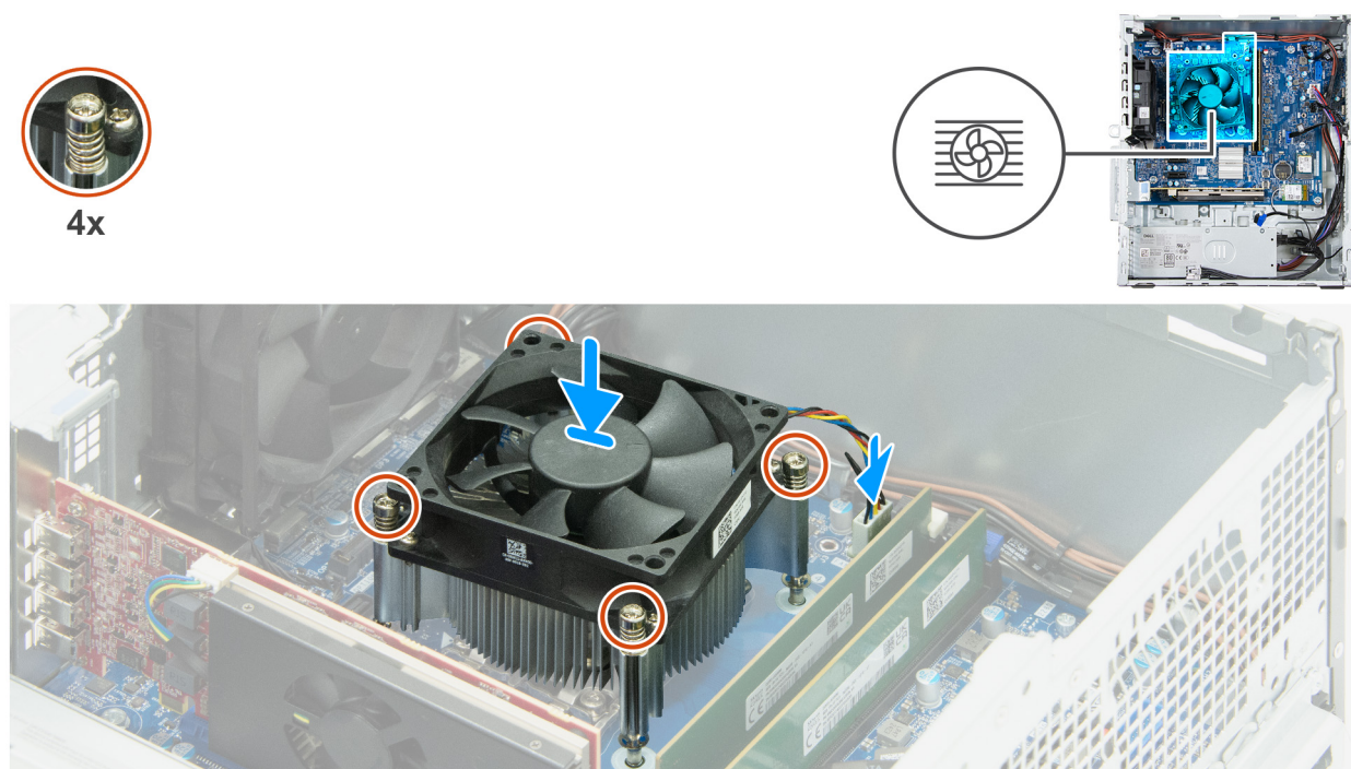
Figura 51. Installazione del gruppo ventola del processore e dissipatore di calore
