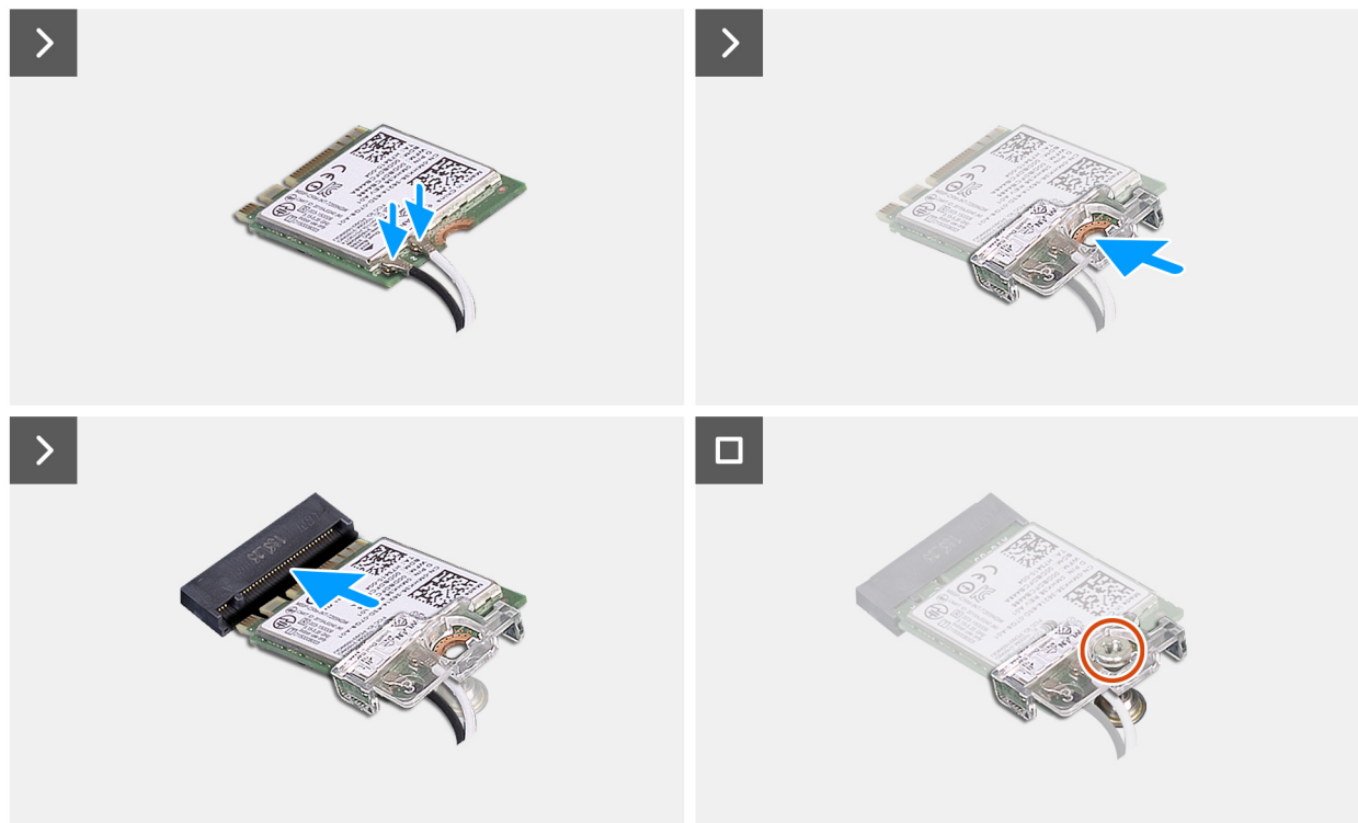
Figura 27. Installazione della scheda wireless
