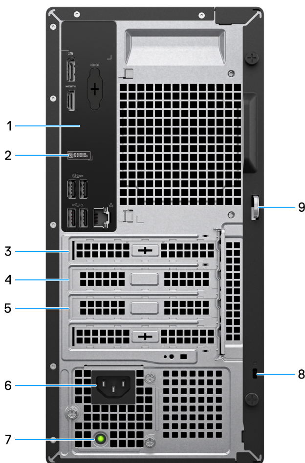
Figura 2. Vista posteriore di Dell Pro Tower Essential QVT1260
