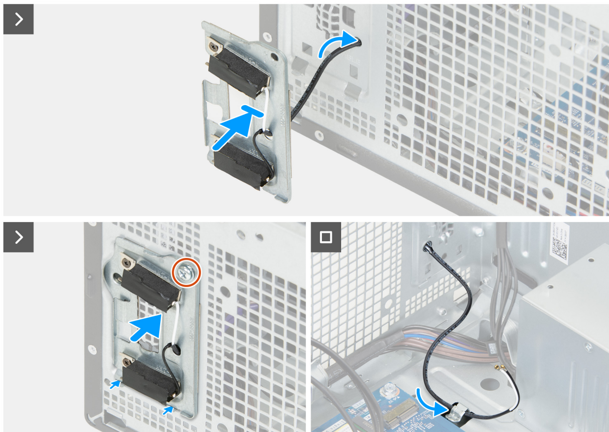
Figura 45. Installazione dei moduli dell'antenna
