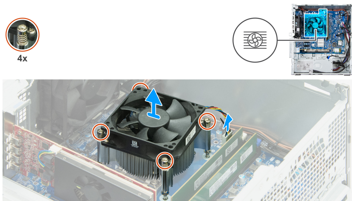
Figura 50. Rimozione del gruppo ventola del processore e dissipatore di calore
