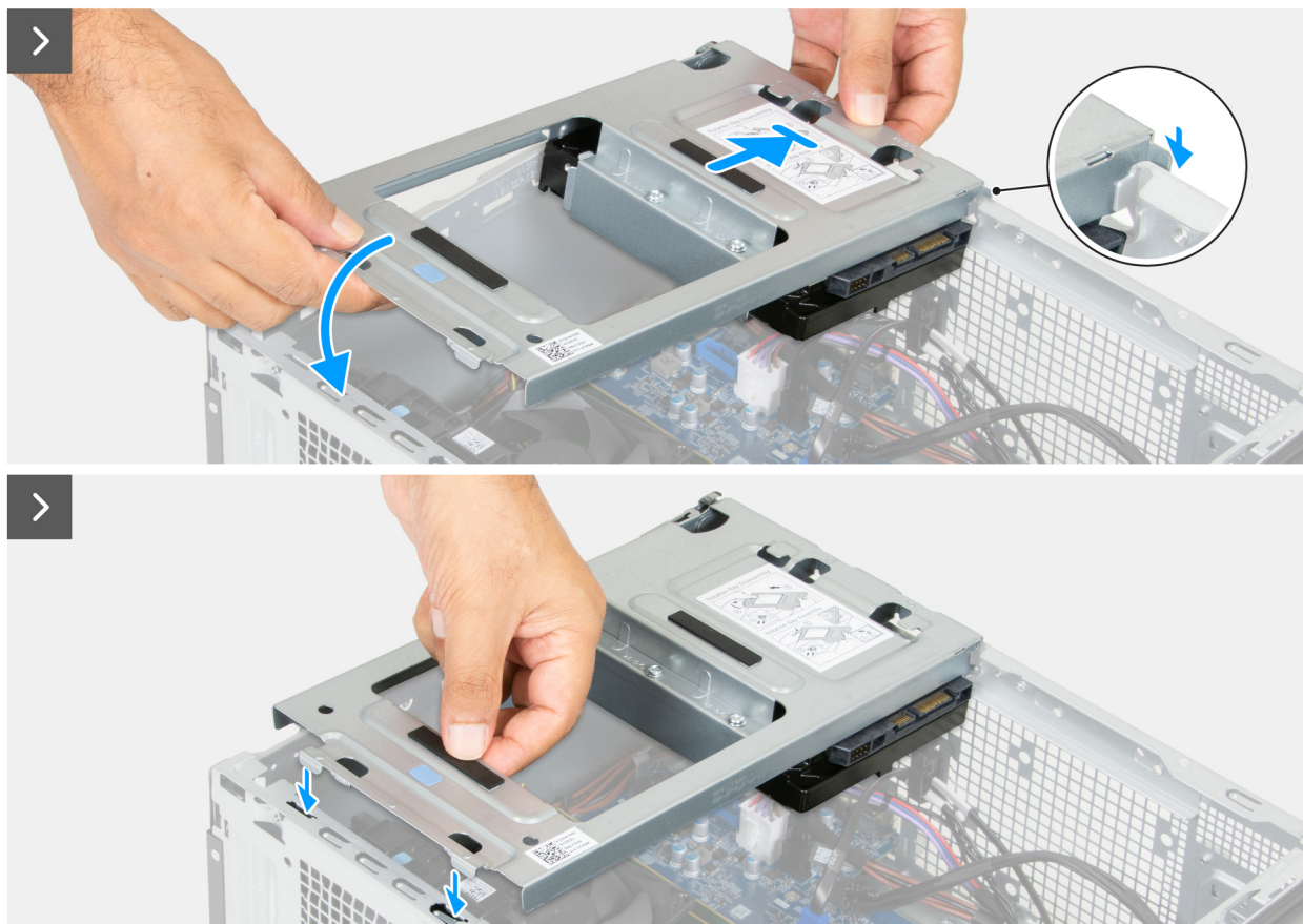
Figura 31. Installazione del drive bay
