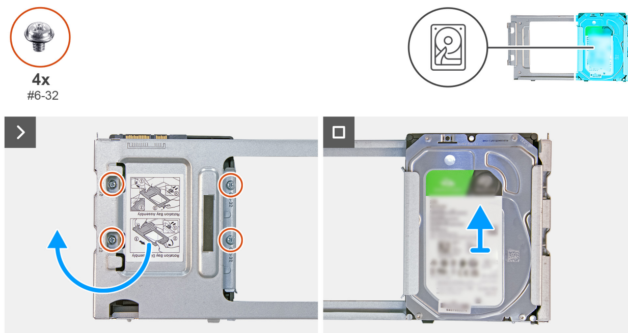
Figura 33. Rimozione del disco rigido.
