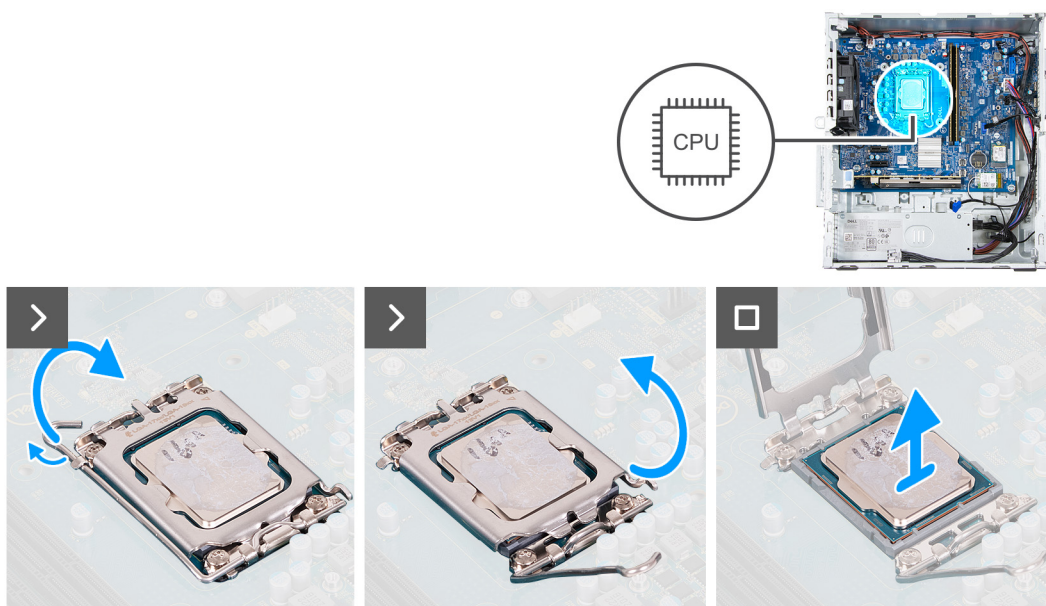
Figura 52. Rimozione del processore
