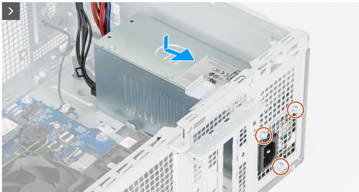
Figura 48. Installazione dell'unità di alimentazione
