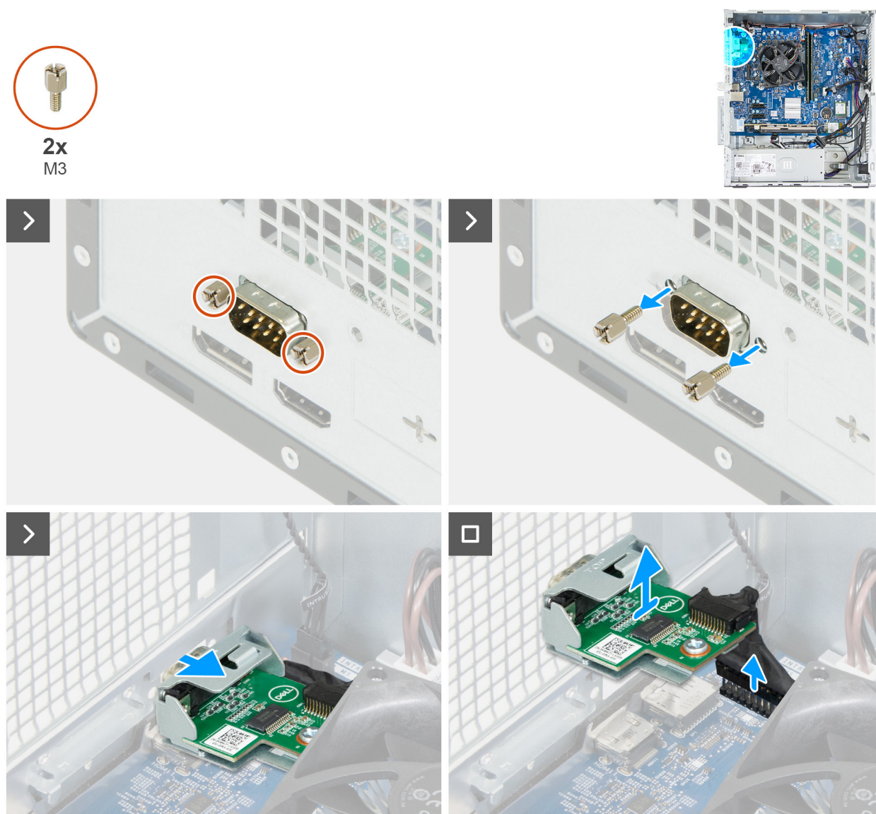
Figura 41. Rimozione del modulo della porta seriale
