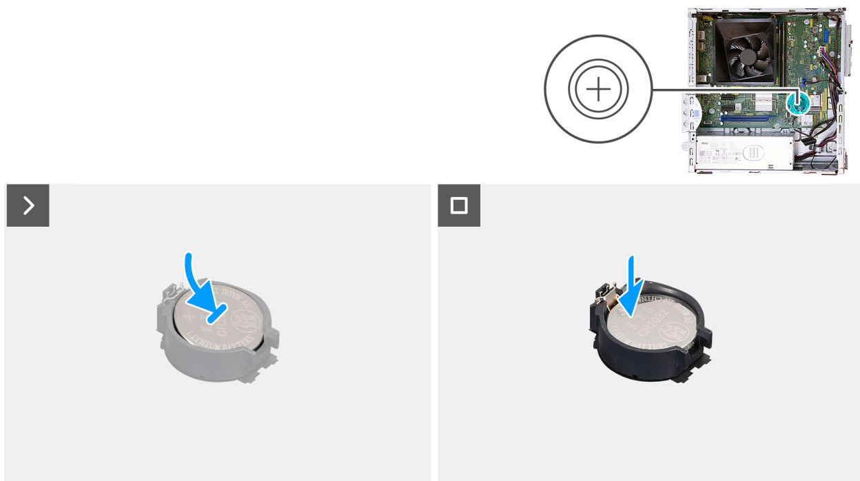
Figura 15. Installazione della batteria a bottone
