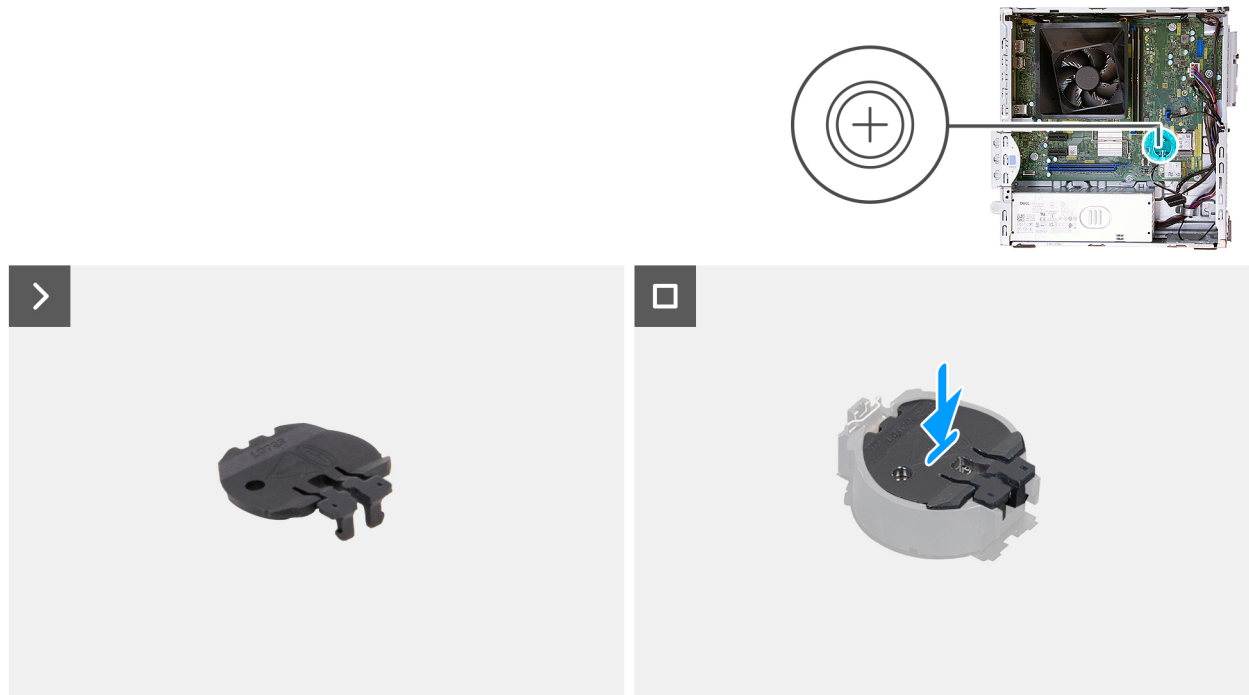
Figura 13. Installazione del coperchio della batteria a bottone
