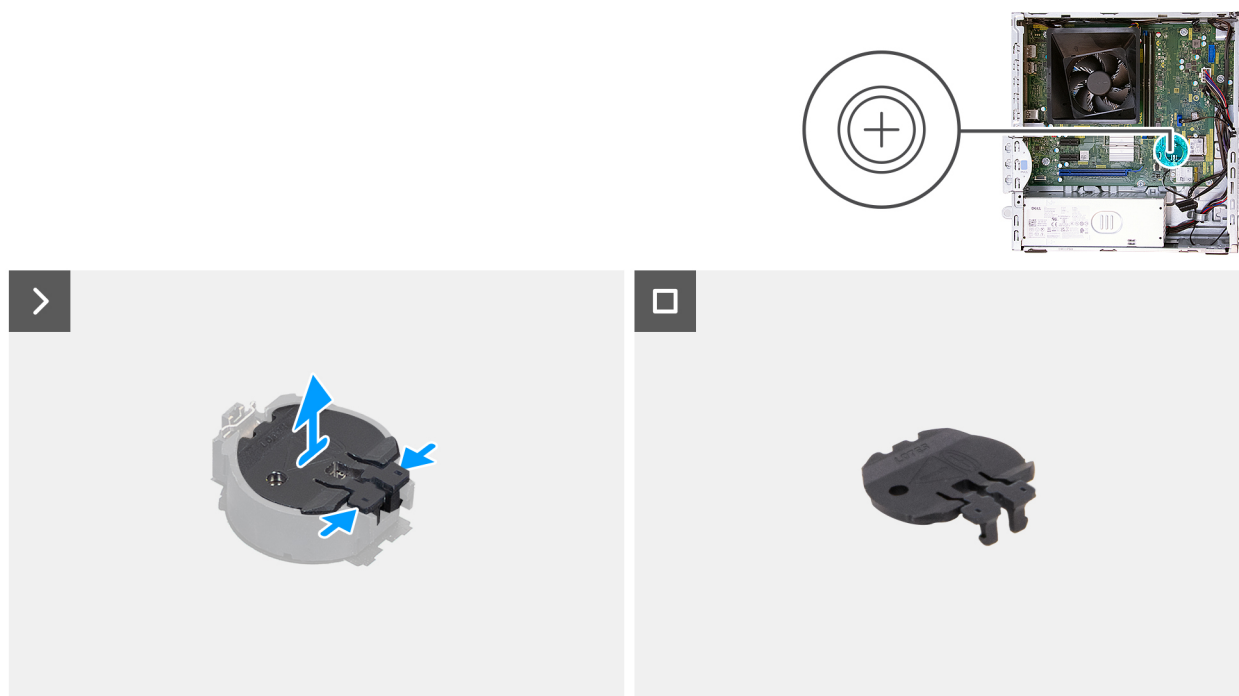
Figura 12. Rimozione del coperchio della batteria a bottone
